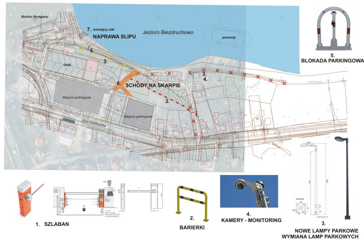
POPRAWA BEZPIECZEŃSTWA NA TERENIE POBIEDZISK - REJON KĄPIELISKA PRZY JEZIORZE BIEZDRUCHOWO KONCEPCJA
